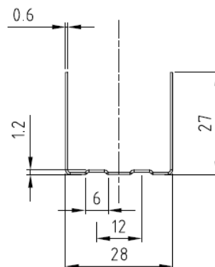
Desen tehnic UD30
